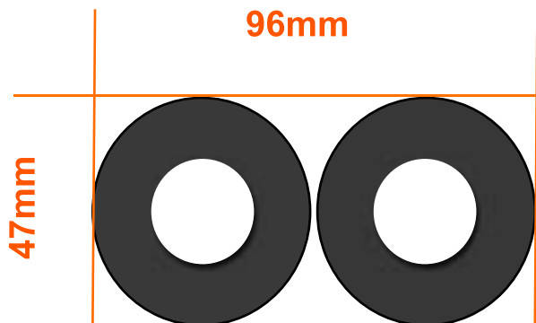
Doppelrohr DN16 mit 13er Dämmung
