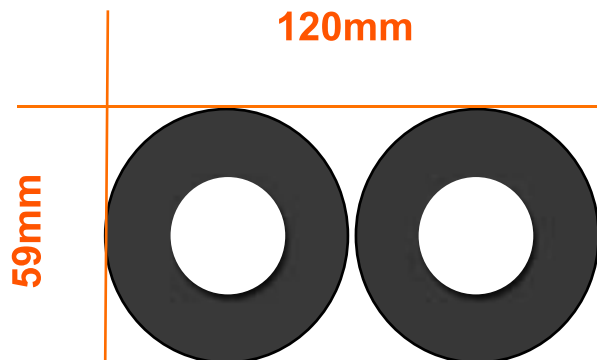
Doppelrohr DN16 mit 19er Dämmung
