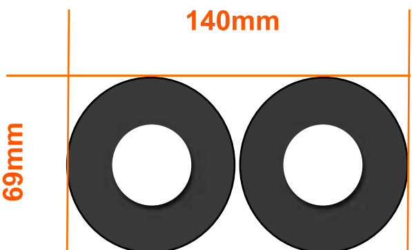
Doppelrohr DN25 mit 19er Dämmung
