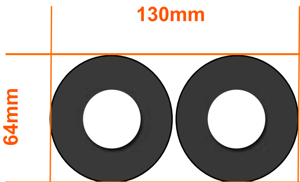
Doppelrohr DN20 mit 19er Dämmung
