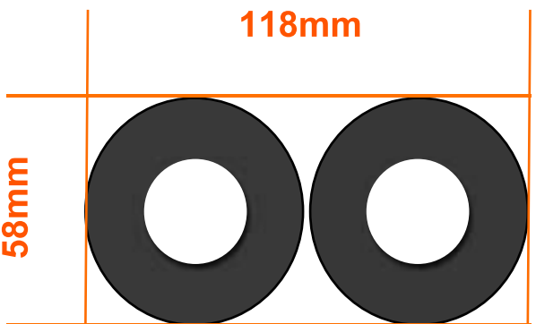
Doppelrohr DN25 mit 13er Dämmung
